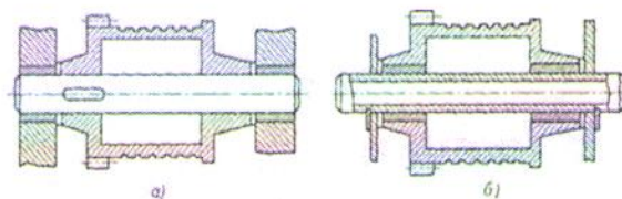
Рисунок 1 – Конструкции осей
